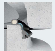
Kombi-Gleitringdichtung SDVseal
